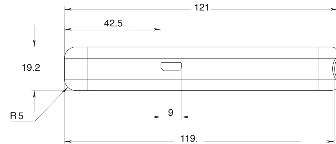
Bottom
